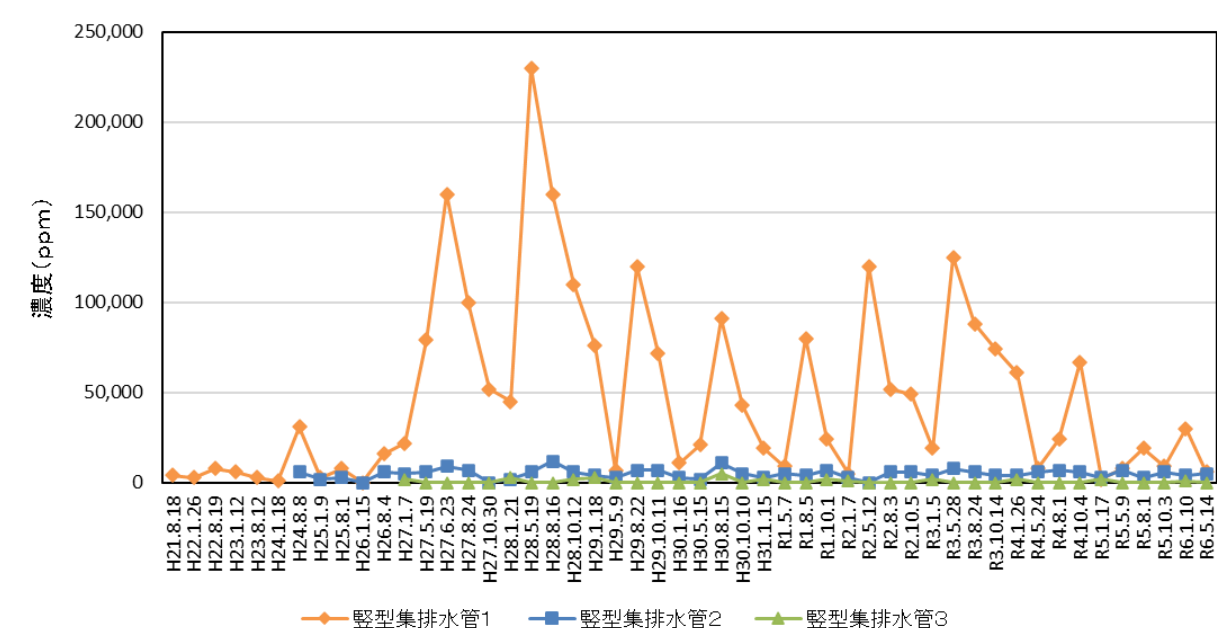
二酸化炭素
