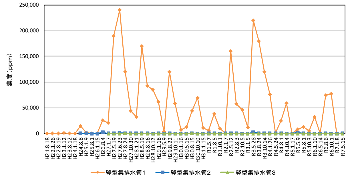
メタン
