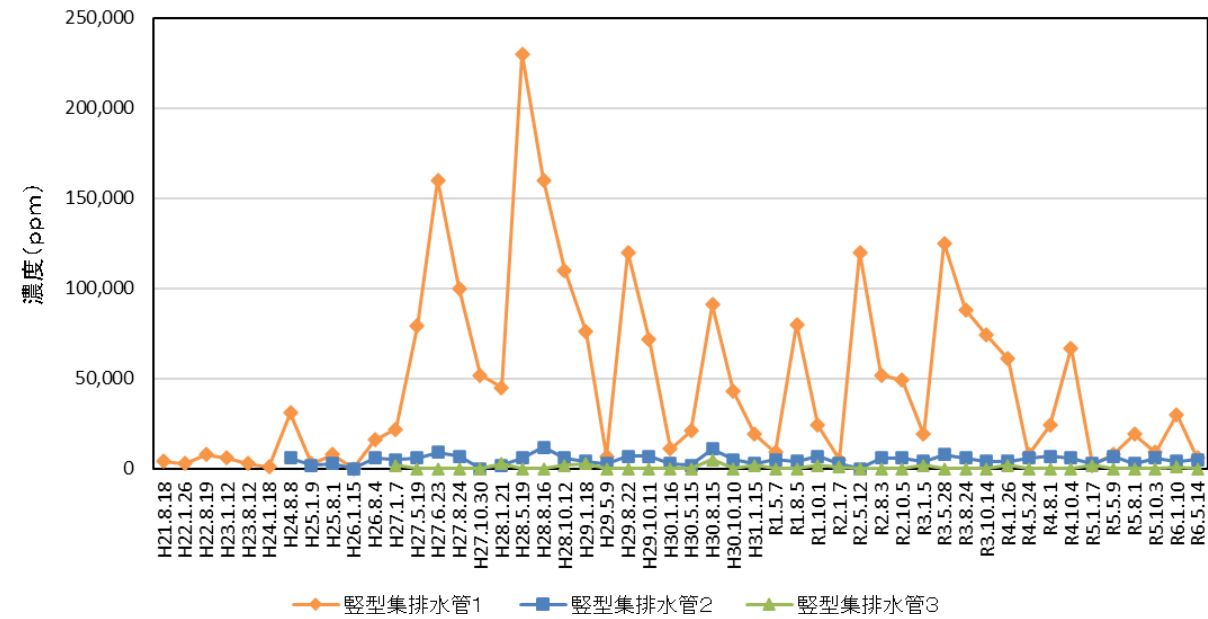
二酸化炭素
