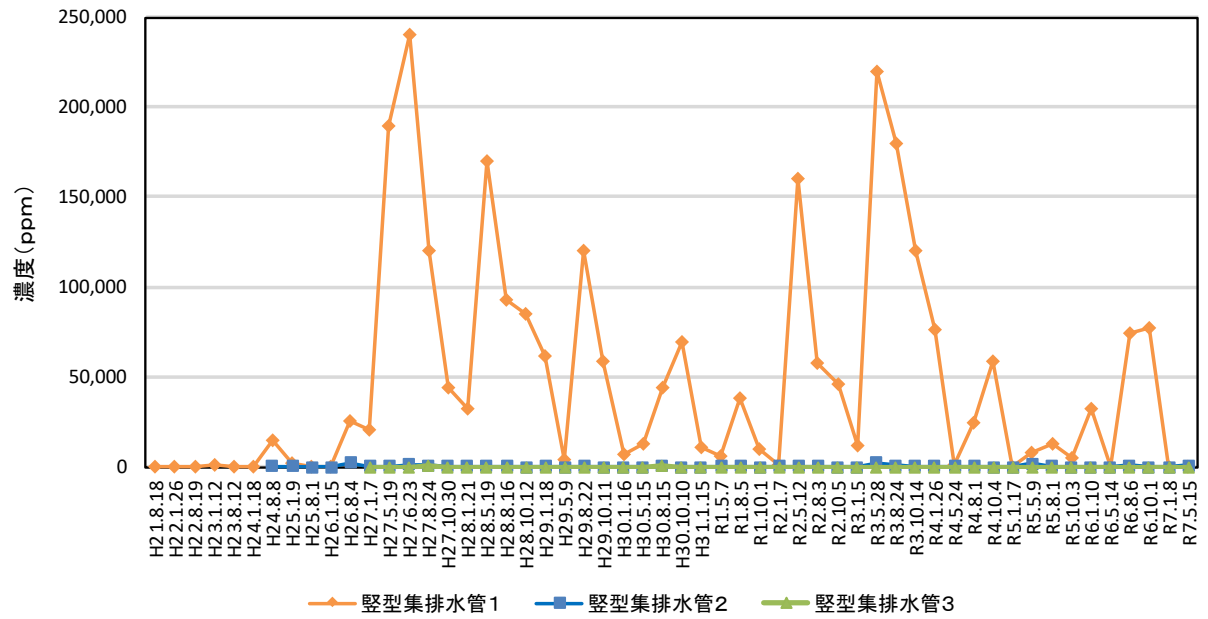
メタン
