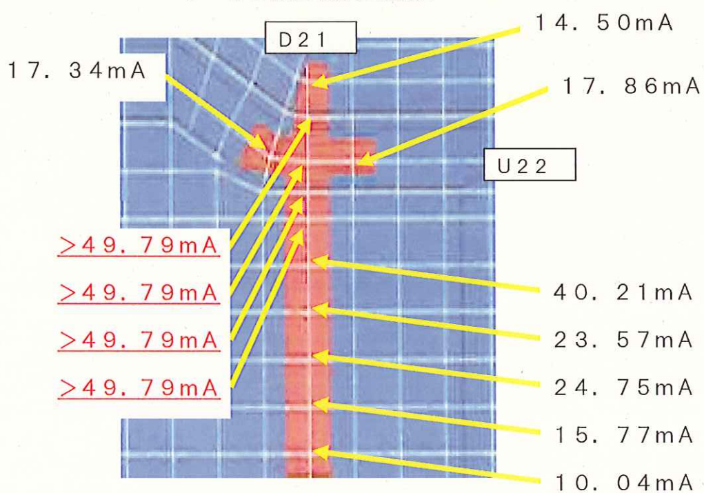
レベル2判定地点の電流値
