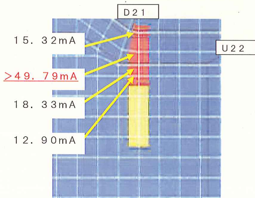
レベル2判定地点の電流値
