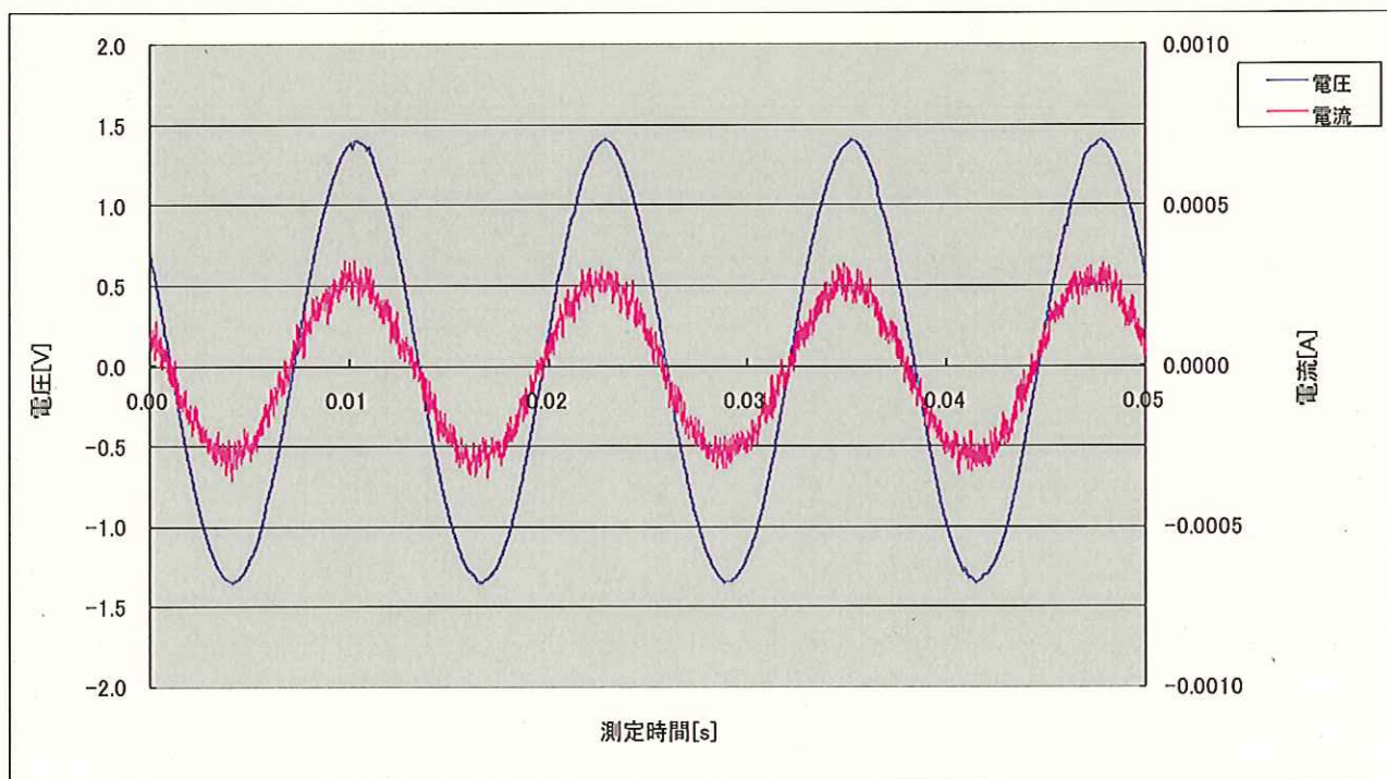
図 7 : 測定時間 : 1 4 時 4 9 分 測定条件 : 1 V、8 0 H z、1 \Omega 、1 0 k N
