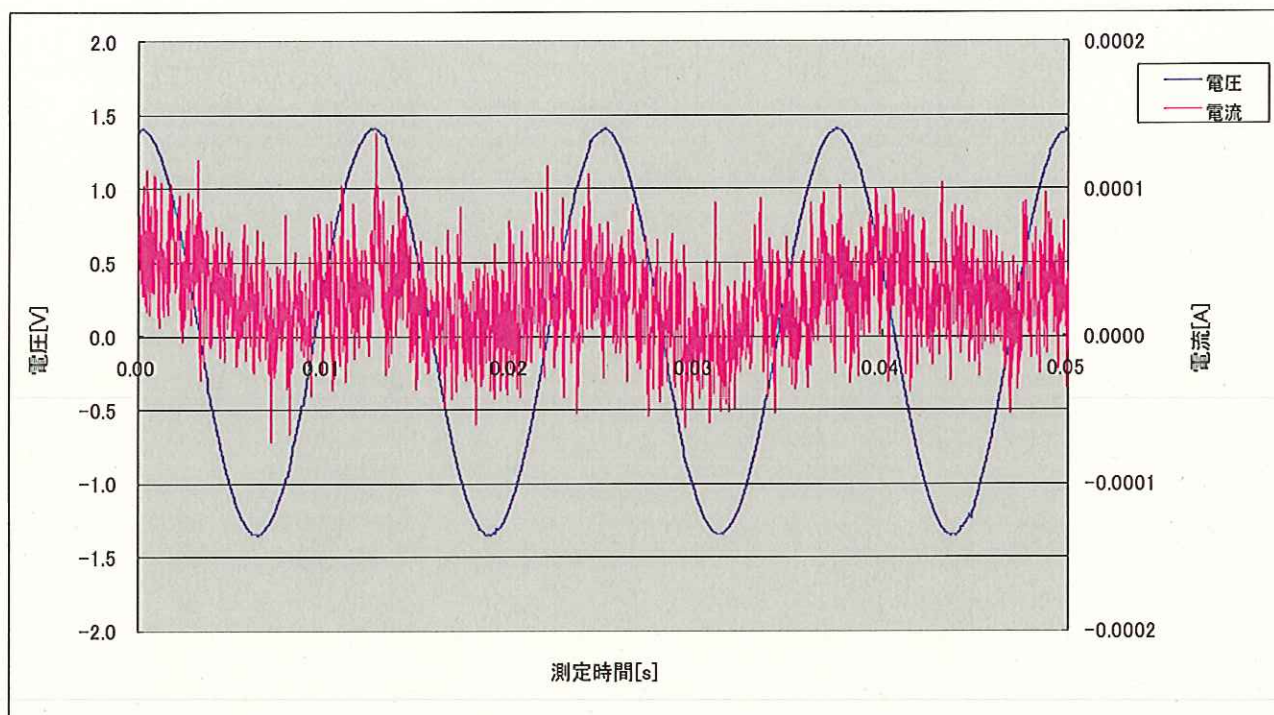
図 6 : 測定時間 : 1 4 時 4 8 分 測定条件 : 1 V、8 0 H z、1 \Omega 、5 k N
