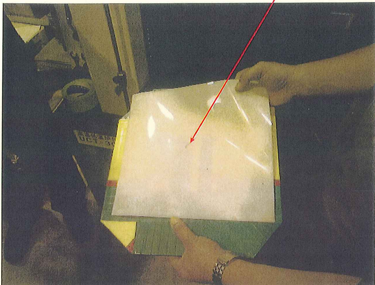
写真-28 実証実験(1日目) 加重面積大で通電なしの上層遮水シートの銅線電極交点部の圧迫跡
