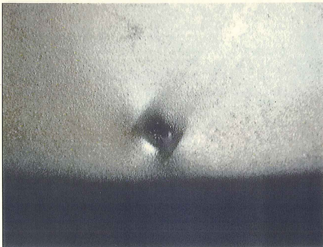
写真-30 実証実験(1日目) 加重面積小で通電ありの上層遮水シートの銅線電極交点部の圧迫跡
