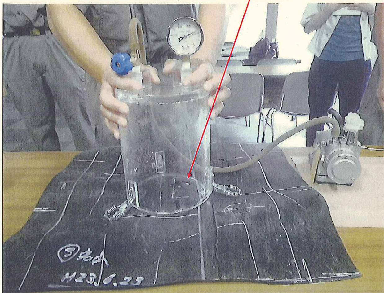
写真-44 実証実験(2日目) ③切り取り遮水シート -25\text{kPa} で気泡発生
