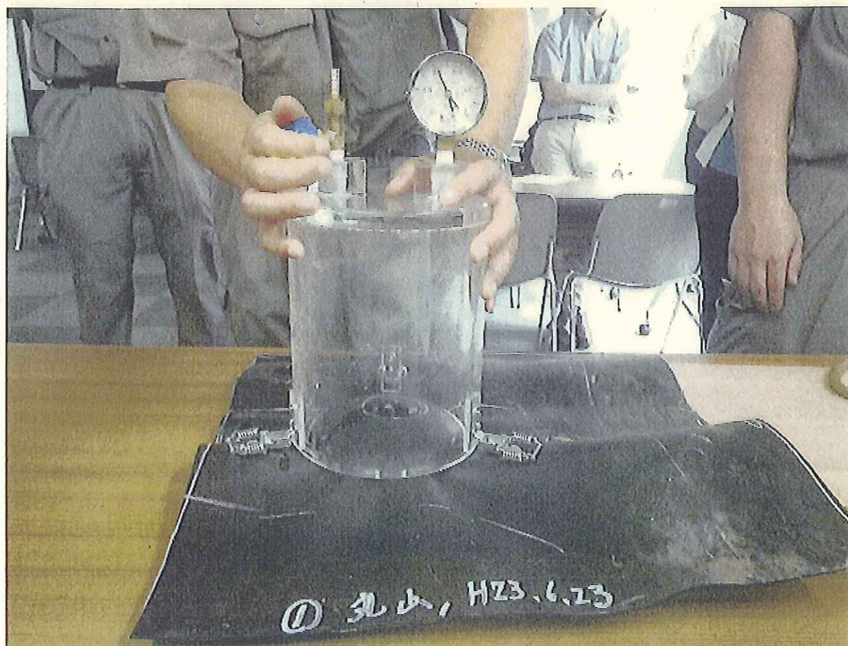
実証実験(2日目) ①切り取り遮水シート -60kPa でも気泡発生なし
