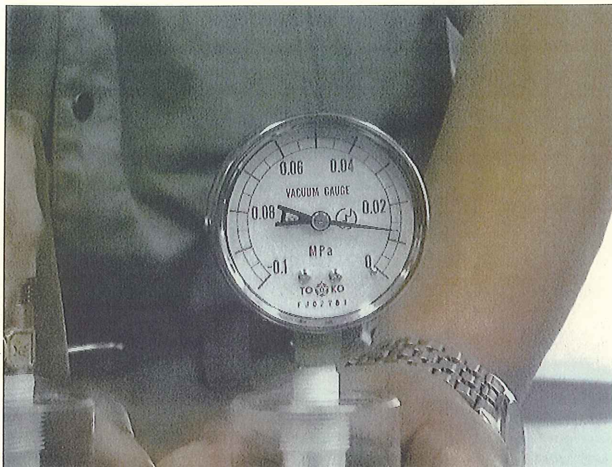
写真-38 実証実験(2日目) 加重面積小で通電ありの2回目では-1kPa未満~-12kPaで気泡発生
