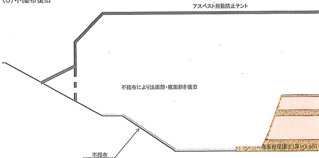
(3)不織布復旧
