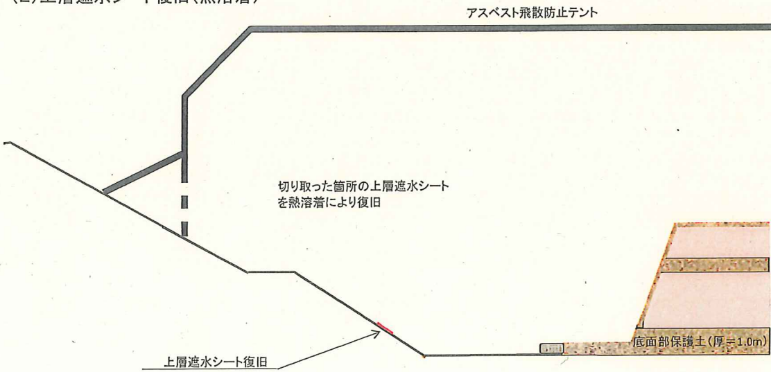
(2) 上層遮水シート復旧(熱溶着)
